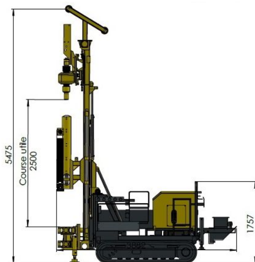
Battage SPT automatique
