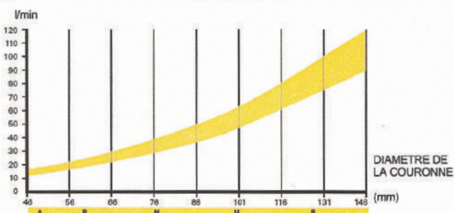
DEBIT D'INJECTION D'EAU (débit recommandé en fonction du diamètre de la couronne)
