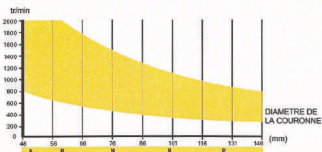
VITESSE DE ROTATION (vitesse recommandée en fonction du diamètre de la couronne)
